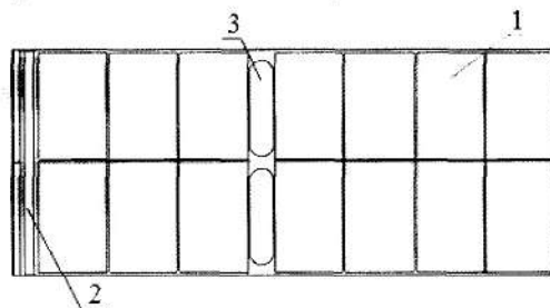
Рисунок 2 - Пример крепления пакетов в продольном направлении с использованием пневмооболочек
