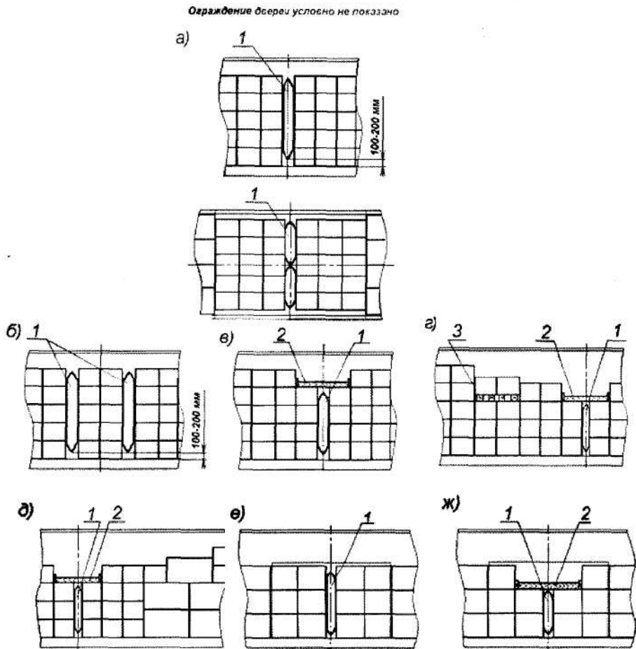
Рисунок 1 – Примеры крепления пакетов в продольном направлении с использованием пневмооболочек
